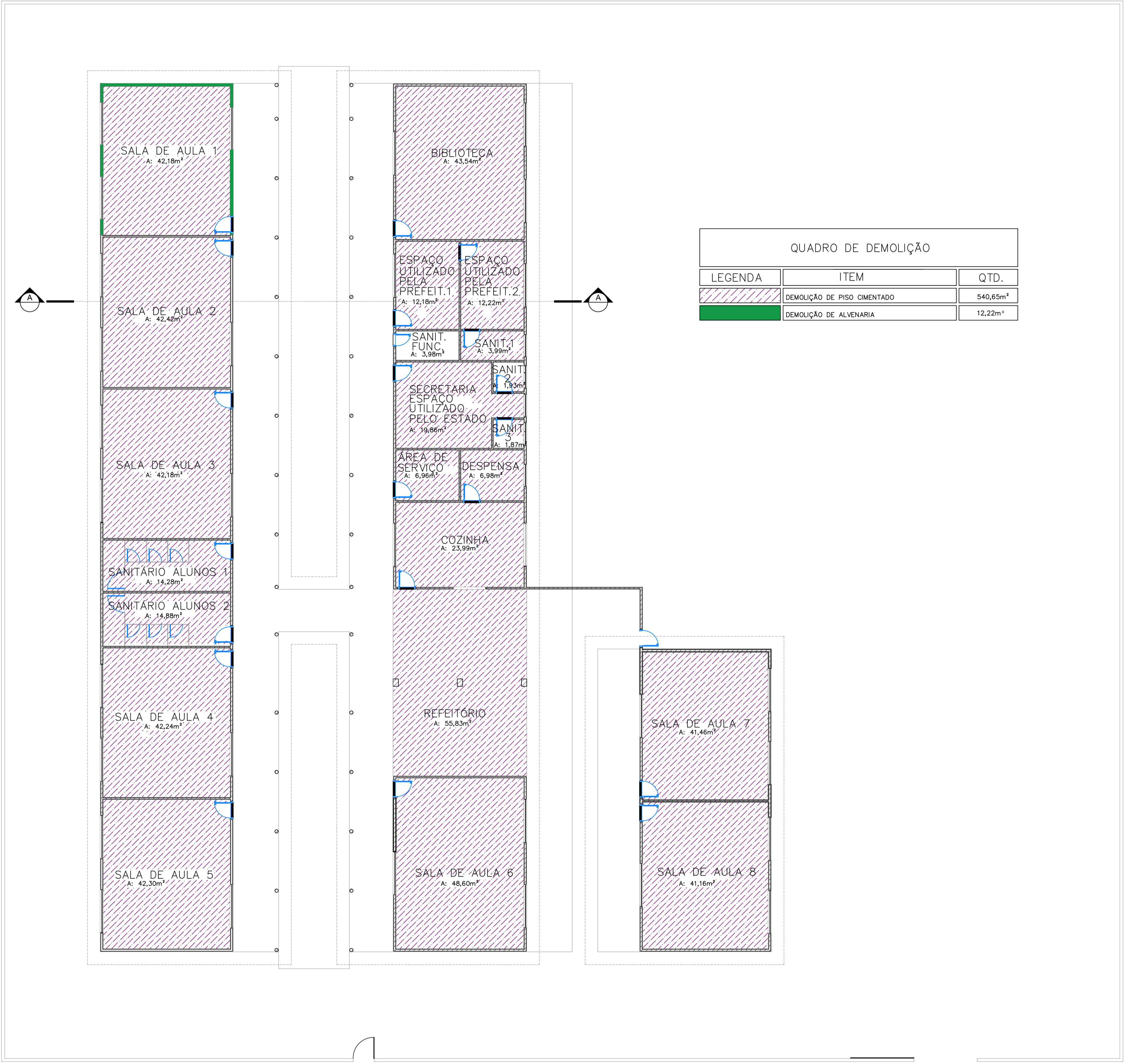
3 PLANTA DE DEMOLIÇÃO ESCALA 1:100
