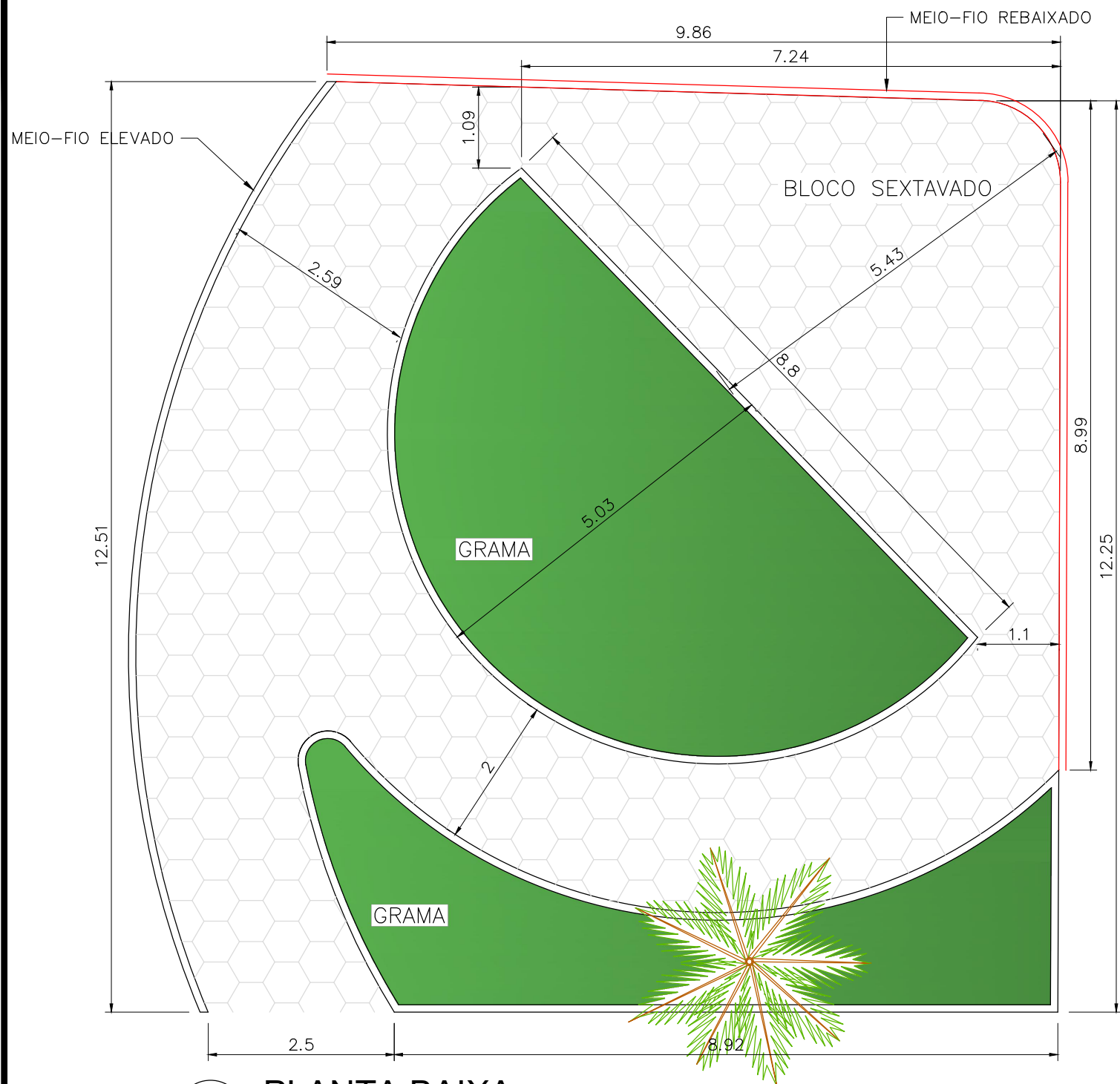
1 PLANTA BAIXA ESCALA 1:75
