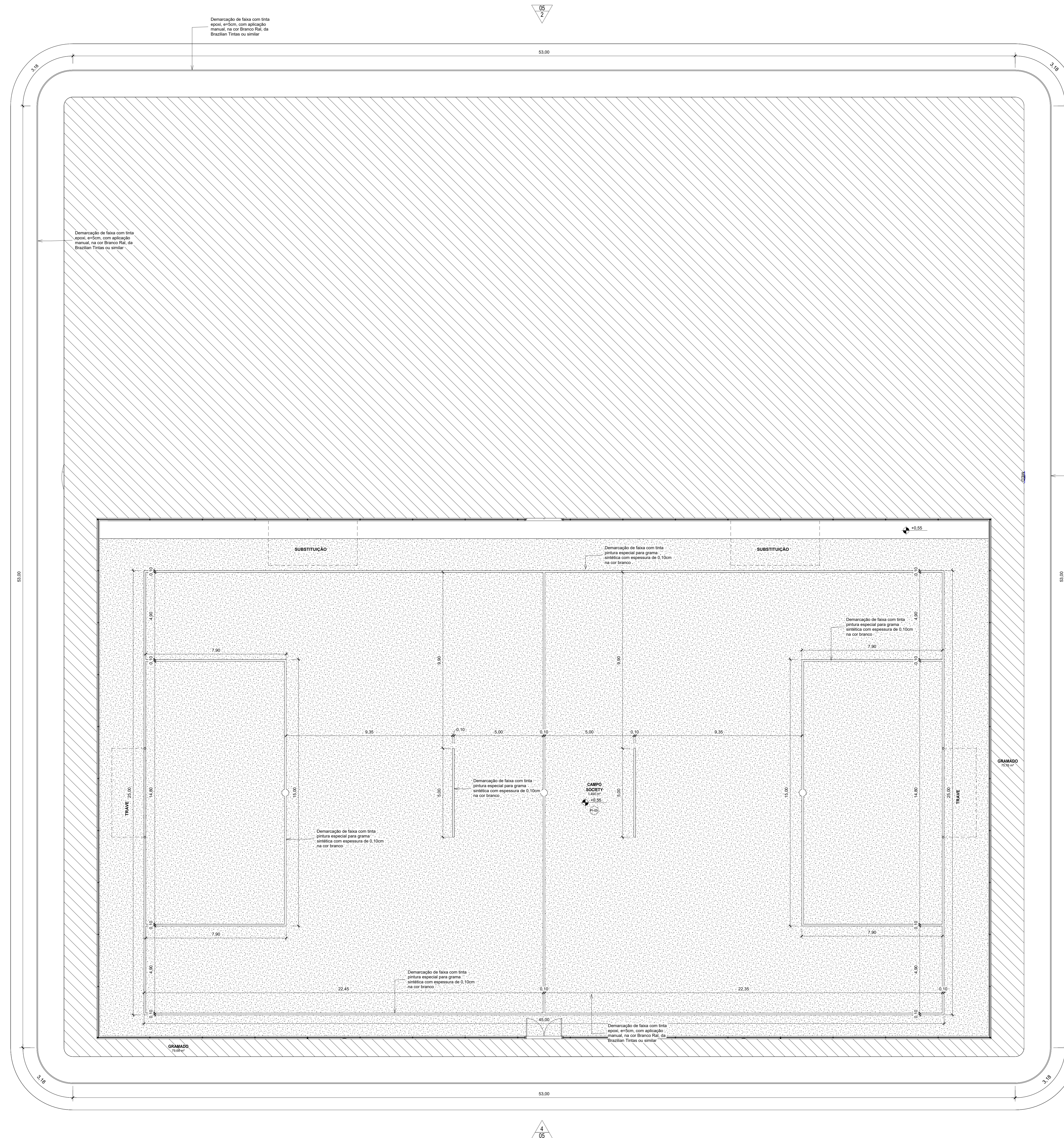
1 Planta Baixa - Marções Campo/Pista 1 : 85
