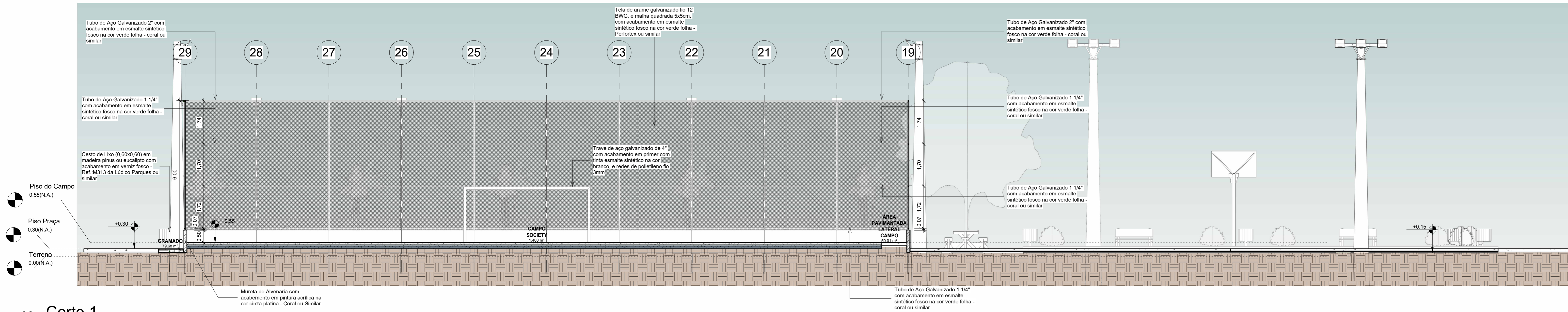
1 Corte 1 1:75
