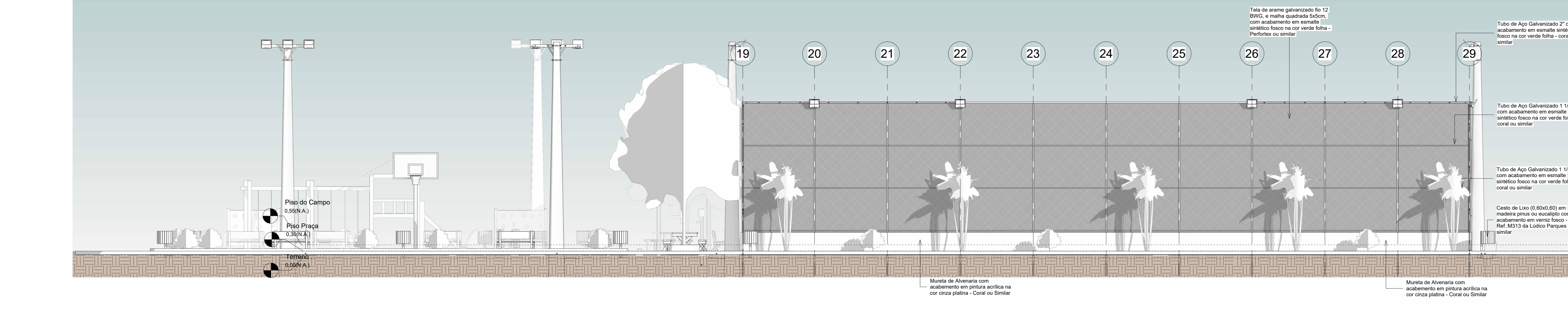
3 Fachada Oeste 1 : 75
