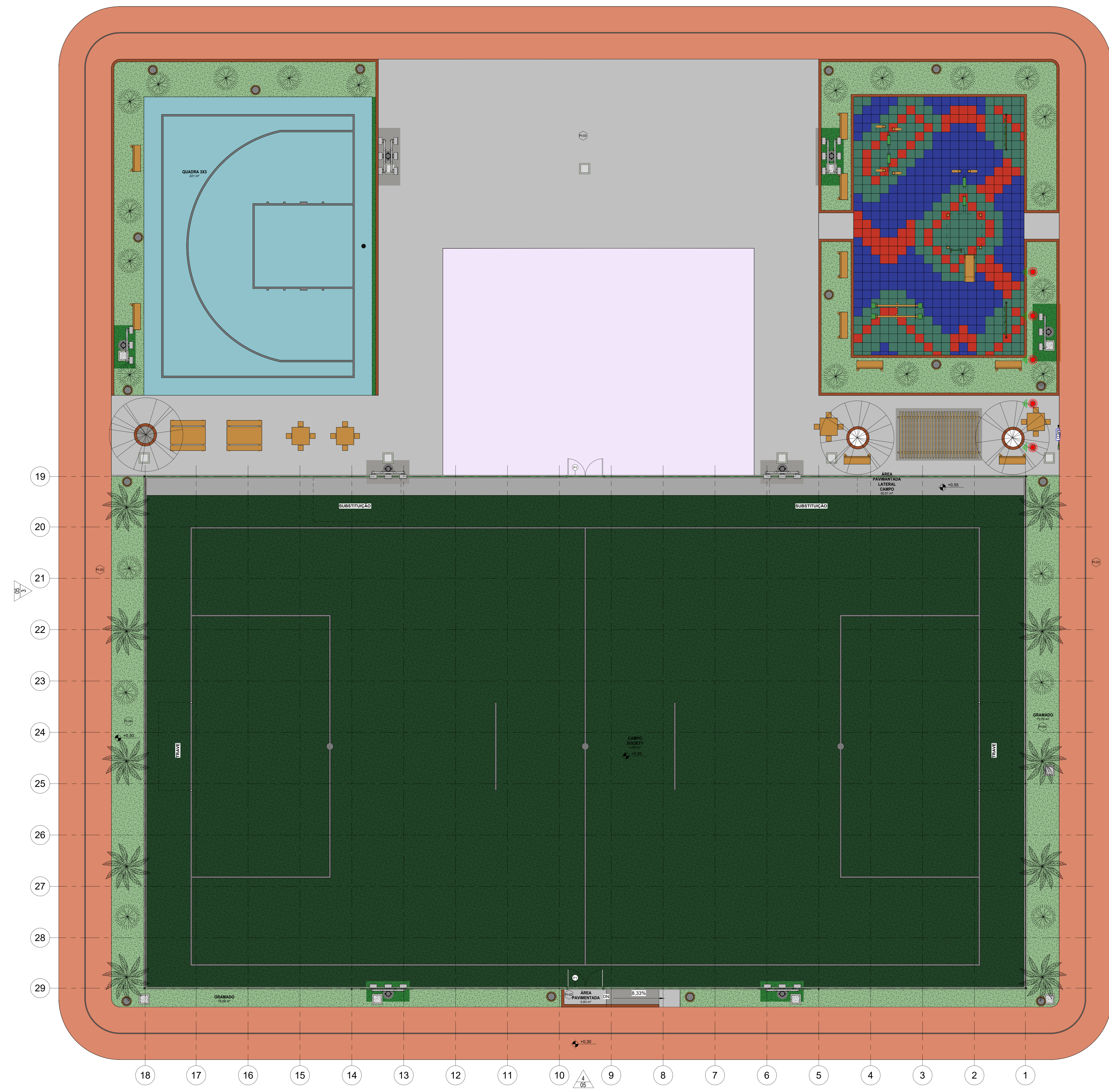
1 Planta Baixa - Layout 1 : 85
